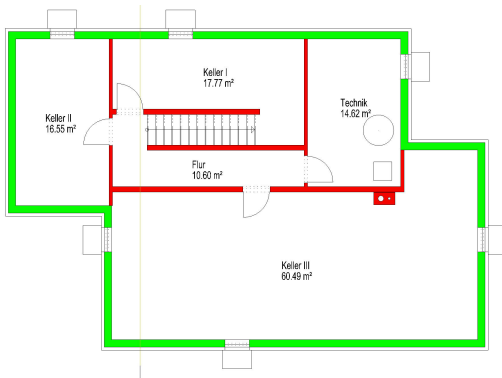
Untergeschoss (Nutzfläche: ca. 120,03 m²)
