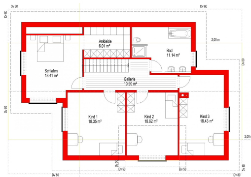
Dachgeschoss (Wohnfläche: ca. 101,86 m²)
