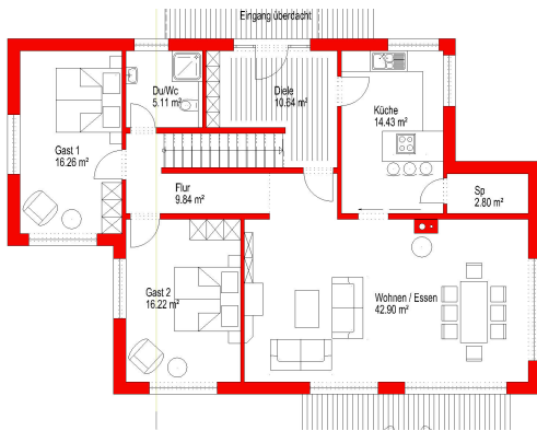
Erdgeschoss (Wohnfläche: ca. 118,20 m²)
